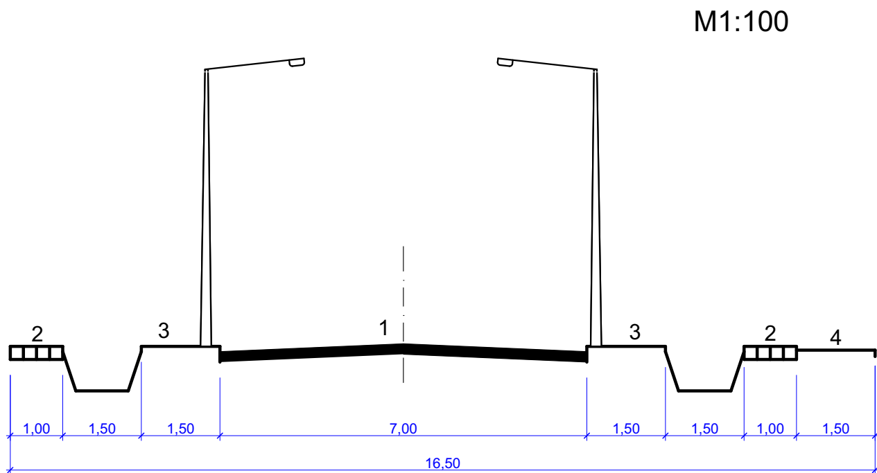
Поперечний профіль дороги виробничого призначення
